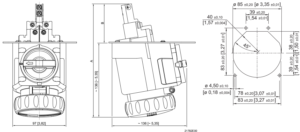
8570/15-4.. 및 8570/15-5.. SolConeX 플랜지 소켓
