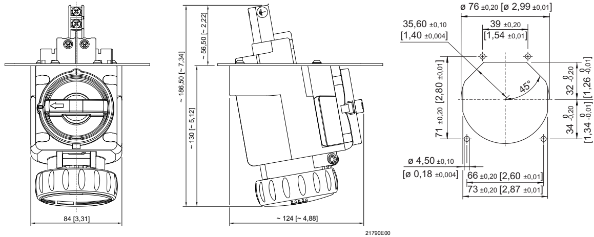
개구부 도면
