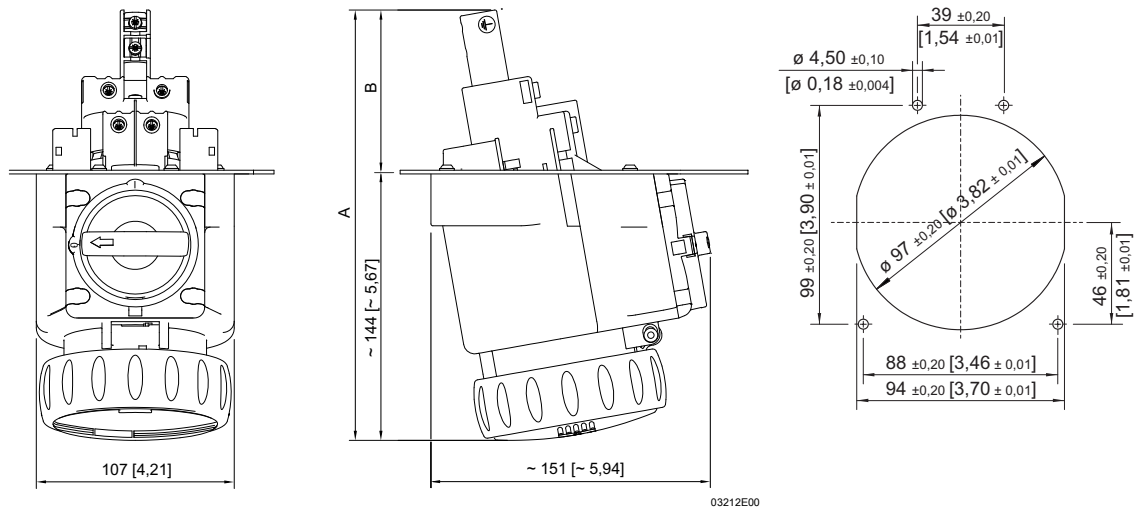
8571/15-4.. e 8571/15-5.. Tomada flangeada SolConeX
