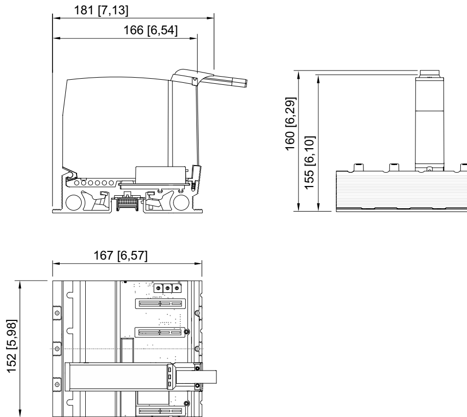
Power Modul V2 9445/35 mit Sockel 9496/35-04
