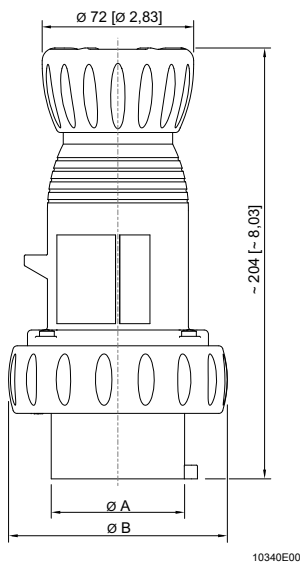
8571/12 Conector SolConeX
