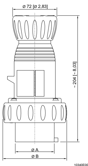
8571/12 Wtyczka SolConeX
