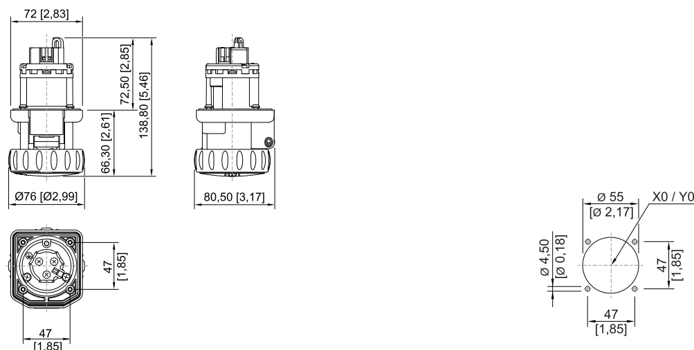
8573/15 SolConeX 低电压法兰插座
