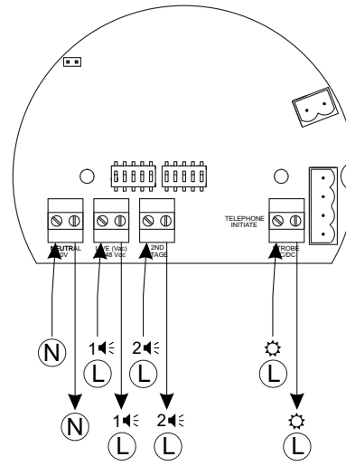
Schaltplan Wechselspannungen
