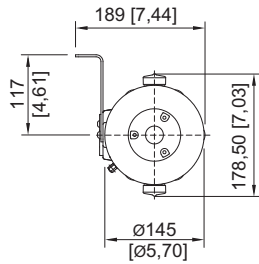
GRP Akustisches Signal Reihe YA6S mit L-Bügel
