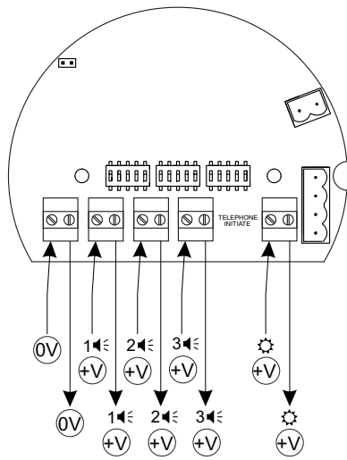
Schaltplan Gleichspannungen
