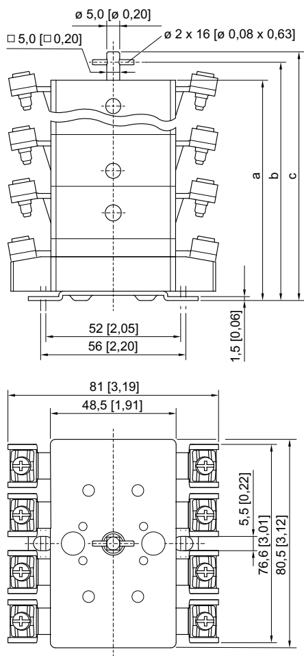
Interrupor de carga e de motor Série 8006/4
