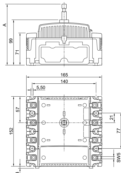
8544/1, 3 pôles + N
