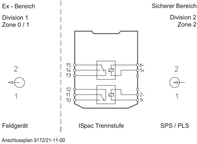
Anschlussplan 9172/21-11-00
