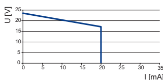
Ausgangskennlinie 9475/32-08-62, 9475/33-08-60
