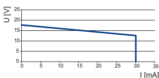
Ausgangskennlinie 9475/32-08-52, 9475/33-08-50
