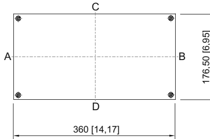
8150/-0360-0176-091-..1.
