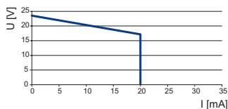
Ausgangskennlinie 9475/32-08-62, 9475/33-08-60
