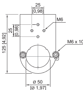
Montageklammer Fläche
