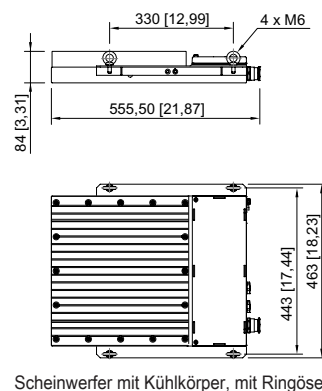
Scheinwerfer mit Kühlkörper, mit Ringösen
