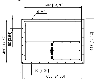
Schalttafel-Einbaumodul Rückansicht
