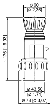
Stecker 3-polig
