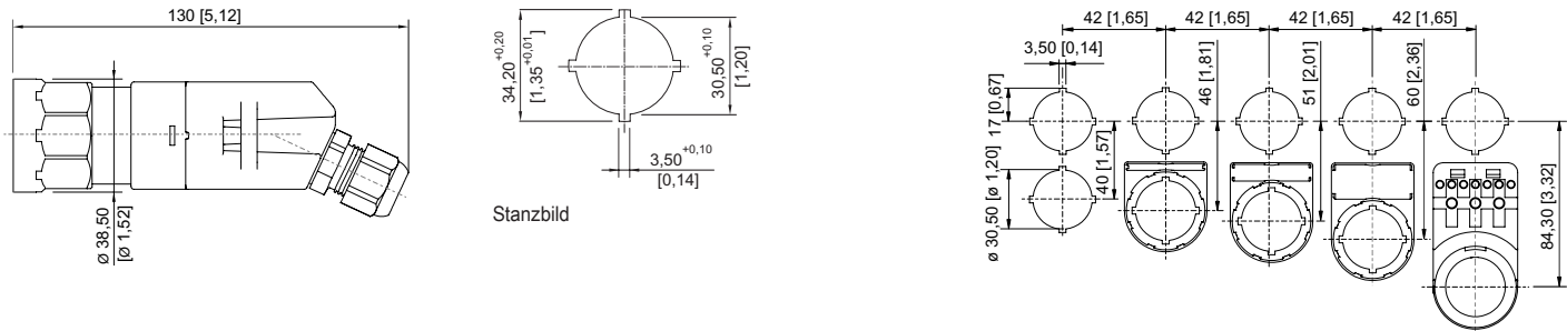
Einbaustermaß mit / ohne Zusatz- Bezeichnungsschild
