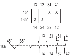
Schaltabwicklung 8008/2-106 Schaltabwicklung 8008/4-11-06
