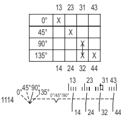
Schaltabwicklung 8008/2-1114 Schaltabwicklung 8008/4-11-114
