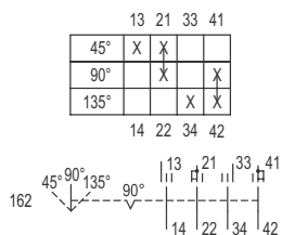
Schaltabwicklung 8008/2-162 Schaltabwicklung 8008/4-11-62
