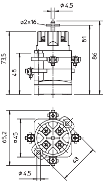
8008/2-6 Lastschalter 3- oder 4-polig
