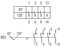
Schaltabwicklung 8008/2-603 Schaltabwicklung 8008/4-16-03
