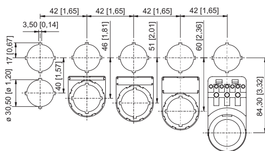
Einbaumaß mit / ohne Zusatz- Bezeichnungsschild
