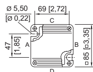
8118/1. Gehäuse Gr. 1
