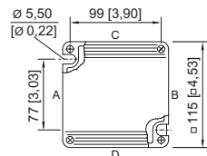
8118/.2. Gehäuse Gr. 2
