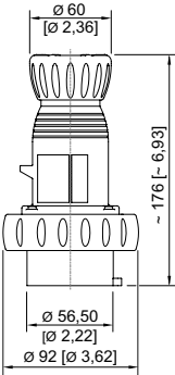
Stecker 5-polig
