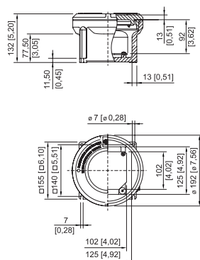
Gehäuse Größe 2 ohne Schauglas
