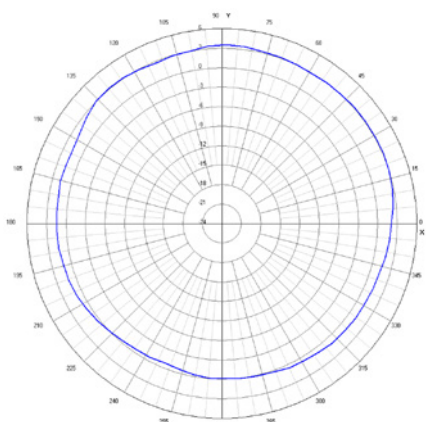
Strahlungscharakteristik für 2,1 GHz Typ 9790/1-0826-NTM-02
