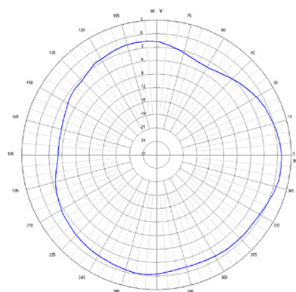
Strahlungscharakteristik für 920 MHz Typ 9790/1-0826-NTM-02
