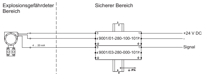
Anwendungsfall: 3 Leiter 4 ... 20 mA Transmitter
