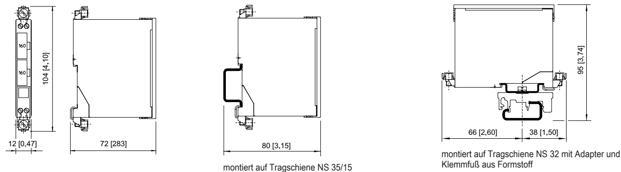
Ein-Kanal-Sicherheitsbarriere für positives Potential
