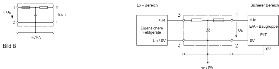
Ein-Kanal-Sicherheitsbarriere für positives Potential
