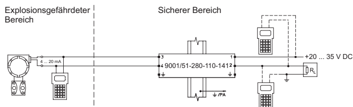
Anwendungsfall: Analogeingang mit Standard-Messumformer Feldstromkreis geerdet
