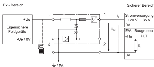
Ein-Kanal-Sicherheitsbarrieren für Messumformer
