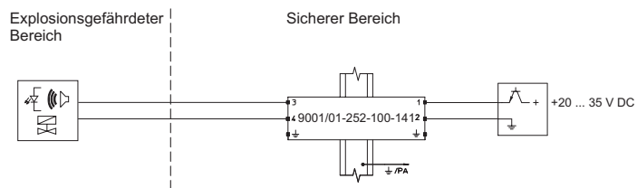
Ein-Kanal-Sicherheitsbarrieren für positives Potential
