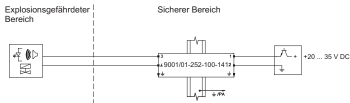
Ein-Kanal-Sicherheitsbarrieren für positives Potential
