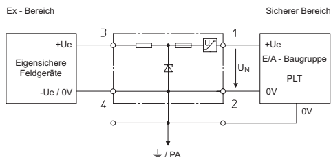
Ein-Kanal-Sicherheitsbarrieren für positives Potential
