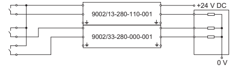
Anwendungsfall: Kombination von potentialfreien Kontakten
