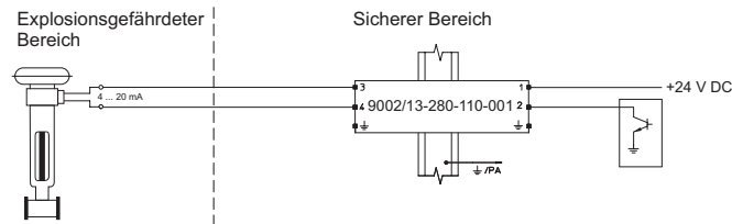
Anwendungsfall: 2-Leiter 4/20 mA I/P Wandler und Stellgeräte - Standard und HART, 4/20 mA Anzeigen
