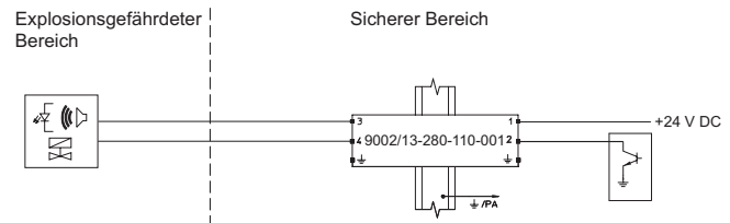
Anwendungsfall: Diskreter 2-Leiter-Ausgang für Magnetventile, LEDs und Signalgeräte
