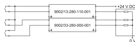
Anwendungsfall: Kombination von potentialfreien Kontakten
