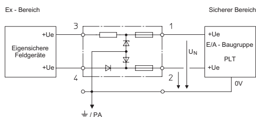
Zwei-Kanal-Sicherheitsbarrieren Sicherheitsbarriere Potential: + / Auswertebatterie Potential: +
