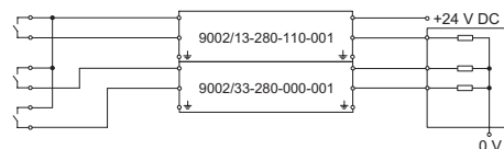
Anwendungsfall: Kombination von potentialfreien Kontakten
