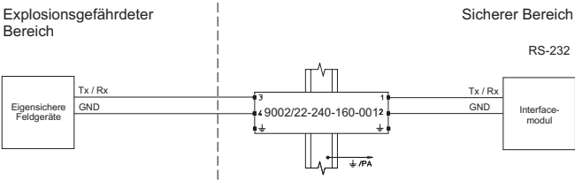
Anwendungsfall mit RS 232
