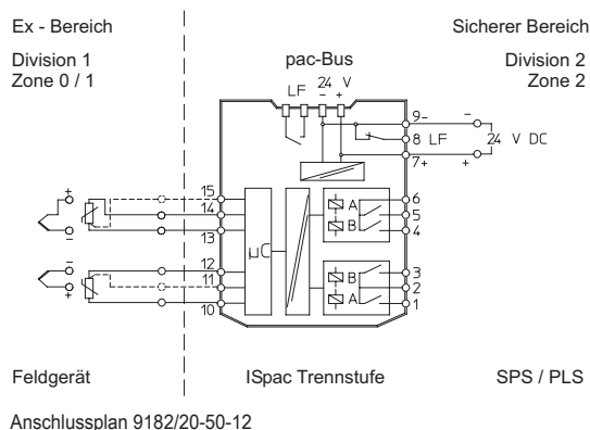
Anschlussplan 9182/20-50-12
