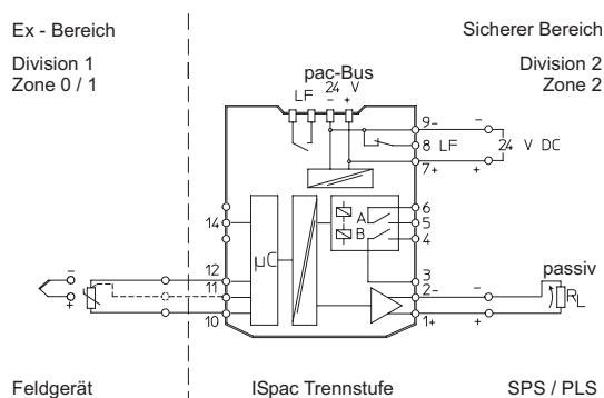
Anschlussplan 9182/10-51-12; 9182/10-51-14
