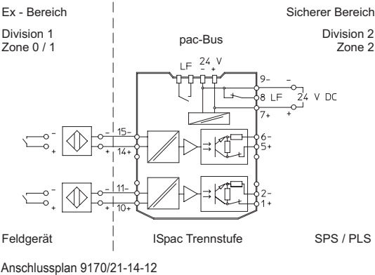
Anschlussplan 9170/21-14-12
