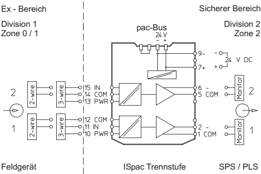
Anschlussplan 9147/20-99-10
