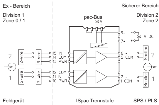
Anschlussplan 9147/20-99-10
