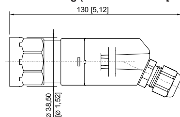
8003/...-726 Drehgriff
