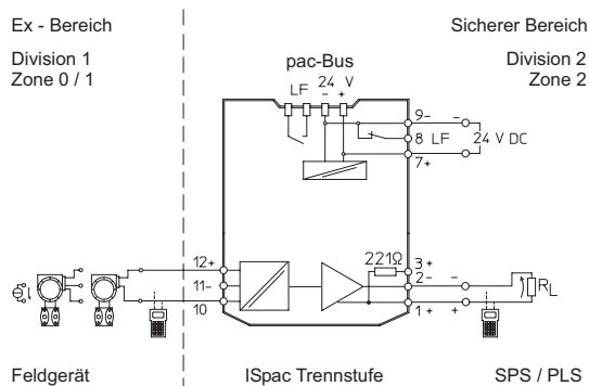
Anschlussplan 9160/13-11-13
