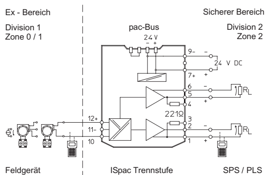
Anschlussplan 9160/19-11-10
