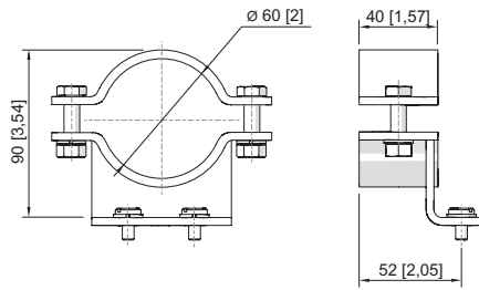
Rohrschelle
