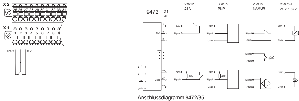
Anschlussdiagramm 9472/35
