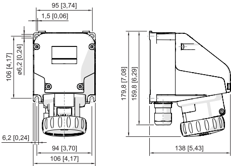
Wandsteckdose kompakt 3-polig
