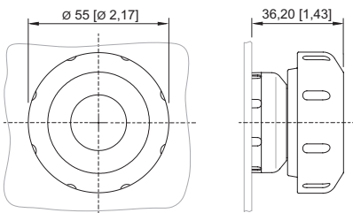
8602/3-014 Pilzdrucktaster rot / schwarz 8602/3-703 Pilzdrucktaster schwarz / schwarz Betätigungsvorsatz mit axialer Betätigung
